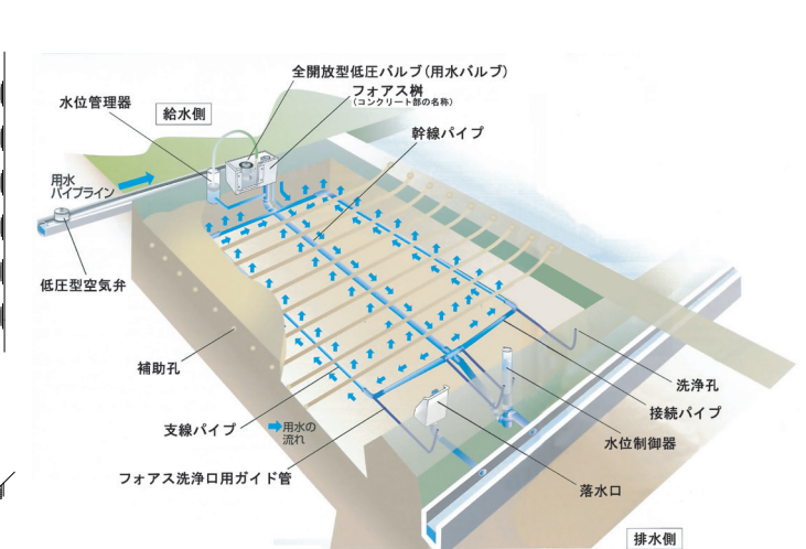
地下水位制御システム「FOEAS」標準図
